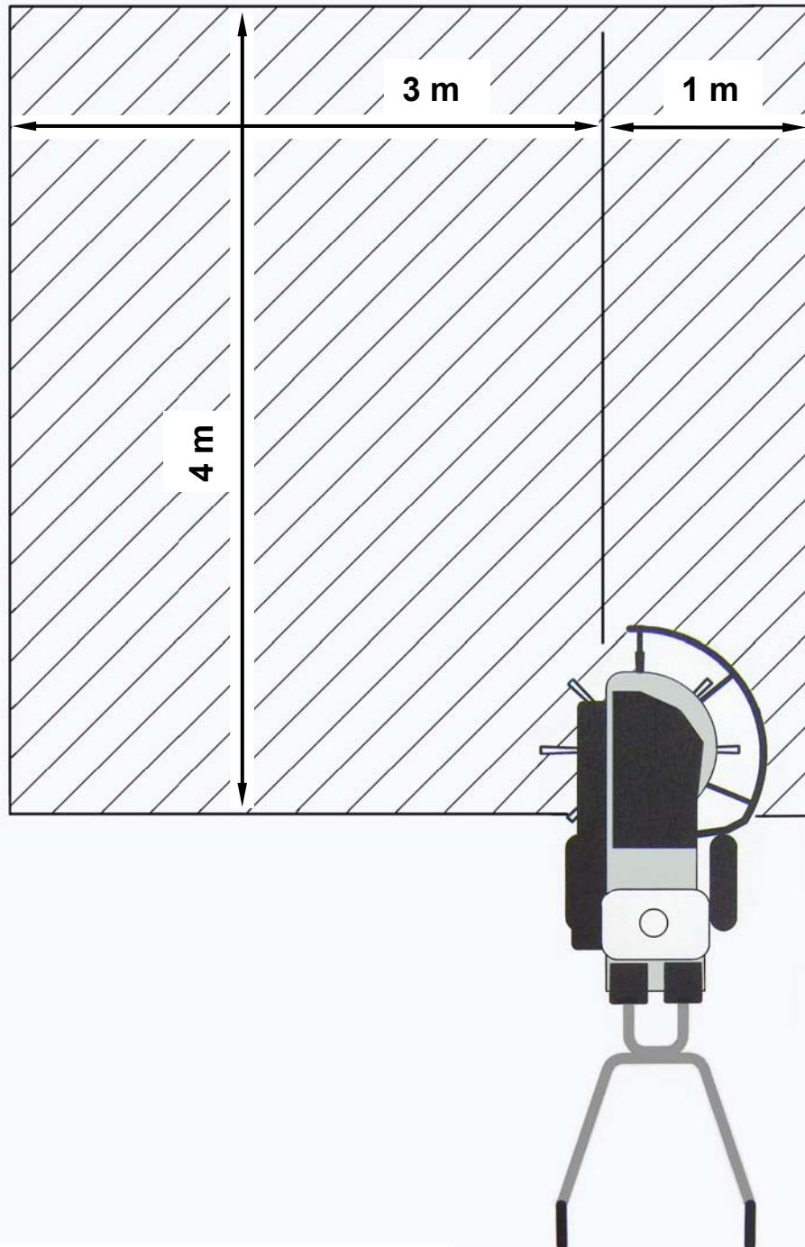
Abbildung 1 : Gefahrenbereich
